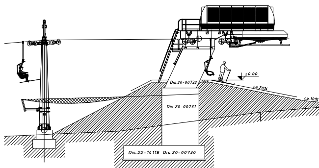
progetto stazione di monte
