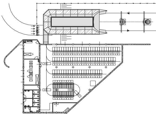
progetto stazione di valle con magazzino veicoli
