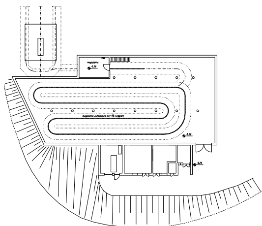
progetto stazione di valle con magazzino veicoli
