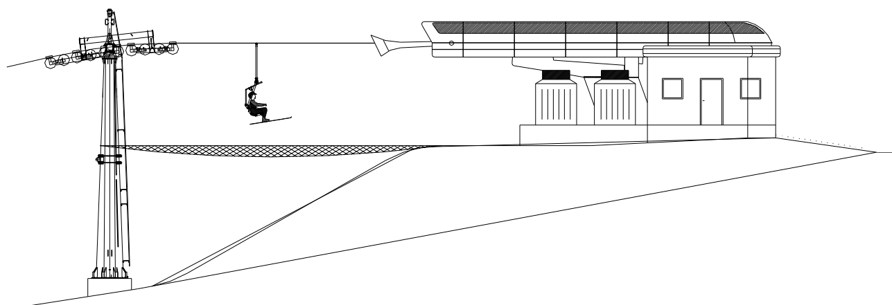
progetto stazione di monte
