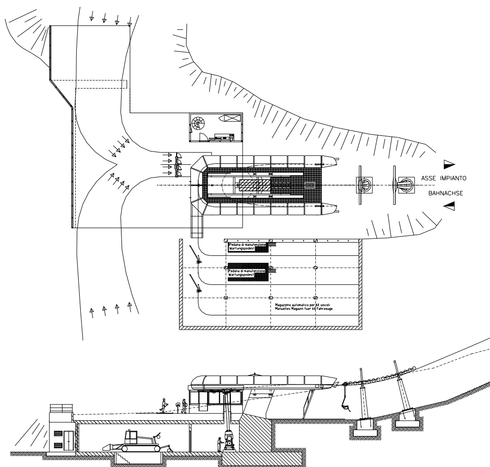
progetto stazione di valle con magazzino veicoli
