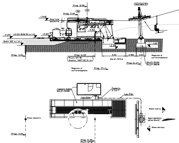
Projekt der Talstation
