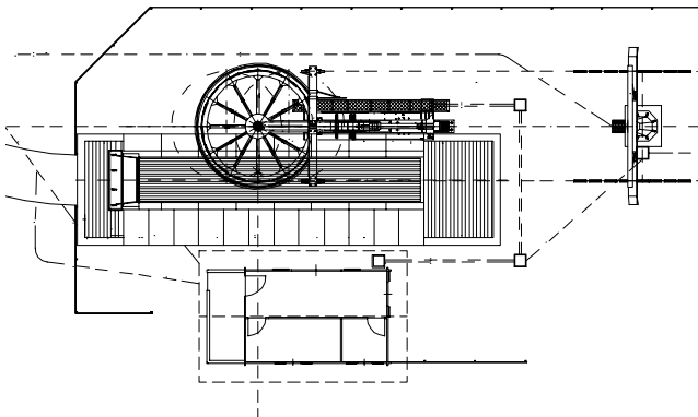
Projekt der Talstation
