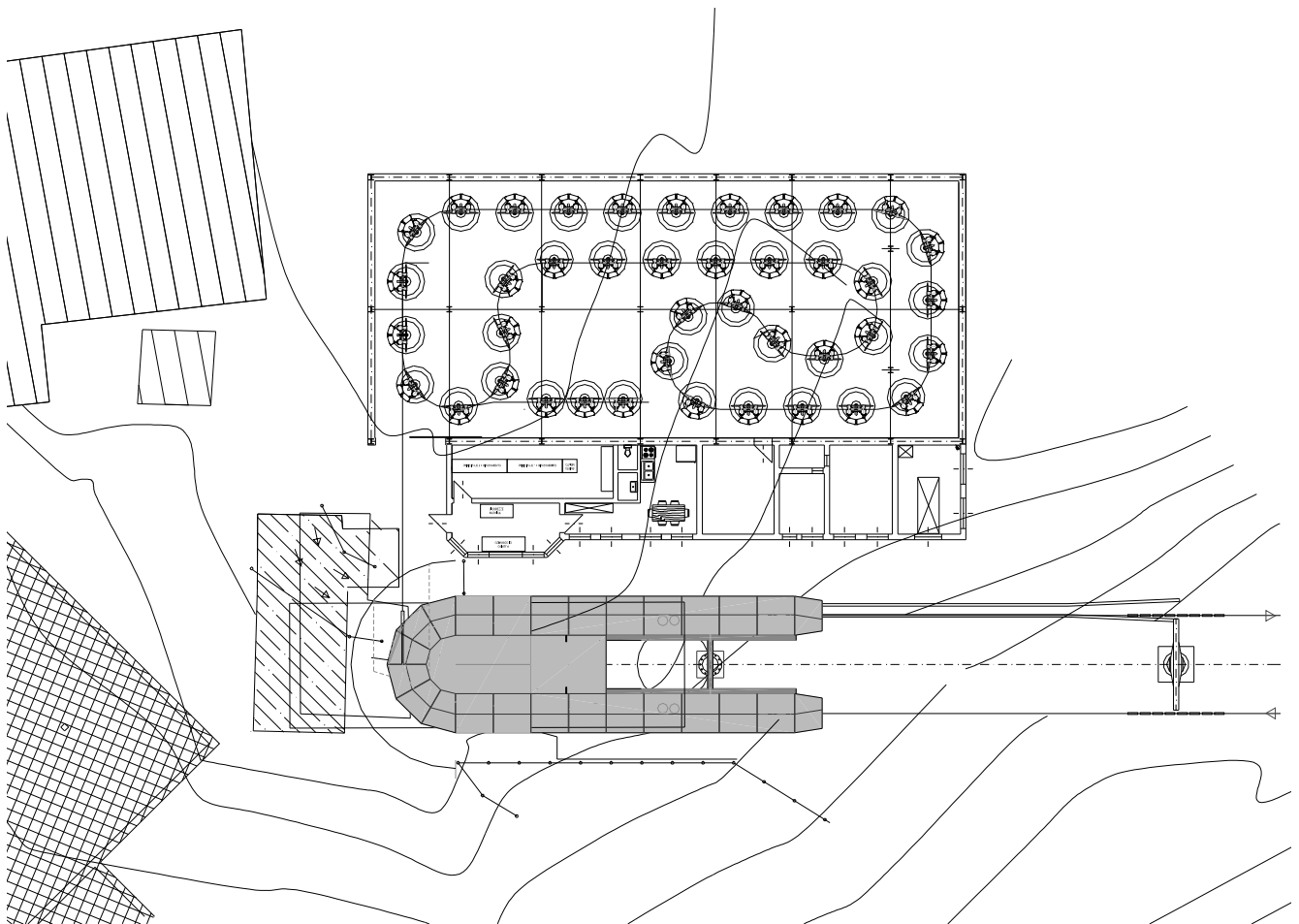
Projekt der Talstation mit Kabinengaragierung
